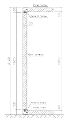
PANEL ESPESOR 80 mm ALTURA TOTAL 2120 mm
